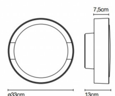
Plaff-on! 33 IP54
