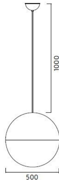
Pendelrör/Pendant tube
